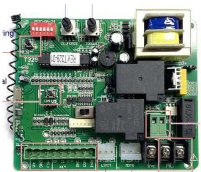
Tarjeta P/Porton
